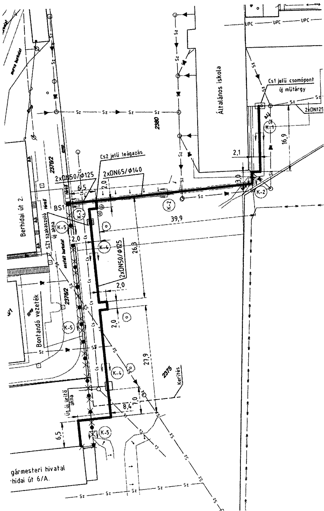
1. kép – Berhidai út 6/A – CS1 csomópont közötti távhővezeték nyomvonal
